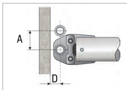
Figura 45 - Distanze minime e ingombro
