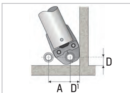
Figura 46 - Distanze minime e ingombro
