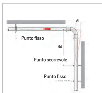
Figura 51 – Compensazione della dilatazione (Bd) con spostamento ortogonale
