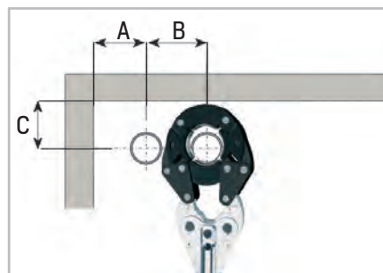
Figura 49 - Quote minime di posa per ganascia avvolgente/catena
