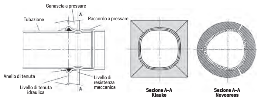
Figura 5 - Vista in sezione di un accoppiamento inoxPRES / steelPRES / aesPRES / marinePRES con catene avvolgenti. Nelle dimensioni \varnothing 42 \div 168,3 mm si ottiene un contorno definito, tipico per ciascun produttore di catene
