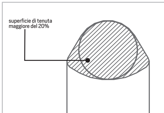
Figura 13 - Profilo dell'anello di tenuta
