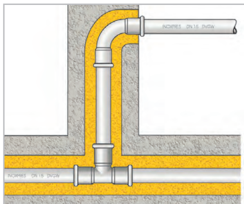
Figura 50a – Creazione di spazi di dilatazione
