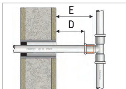
Figura 48 - Distanze minime e ingombro
