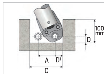
Figura 47 - Distanze minime e ingombro
