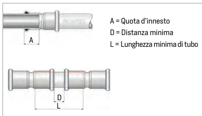
Figura 34 – Quota minima d'innesto ed accoppiamento
