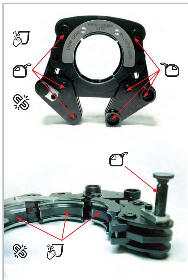
Figura 19 – Attrezzatura Klauke
