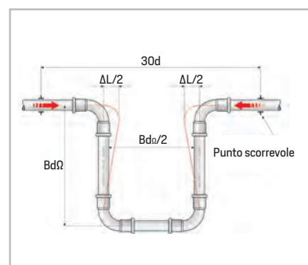
Figura 53 – Compensazione della dilatazione ad U ( Bd\Omega = Bd / 1,8 )
