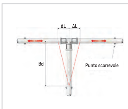
Figura 52 – Compensazione della dilatazione (Bd) mediante stacco a T
