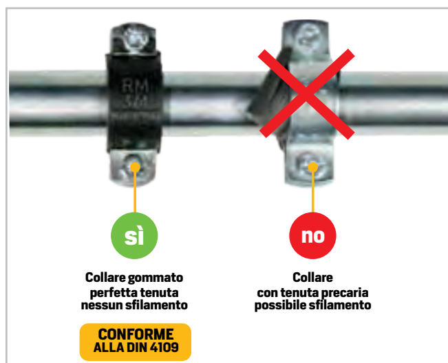
Figura 54 – Collare gommato PRATIKO conforme alla DIN 4109 (articoli RM serie 355/G – 351/G – 555/G – 156/G)
